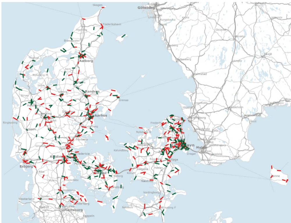
Figur 11 Illustration af Telias (rød) og Telenors (grøn) eksisterende radiokæder i 26 GHz-frekvensbåndet
